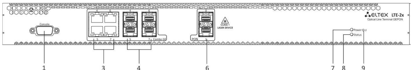
Рисунок 3 – Передняя панель станционного терминала LTE-2X
