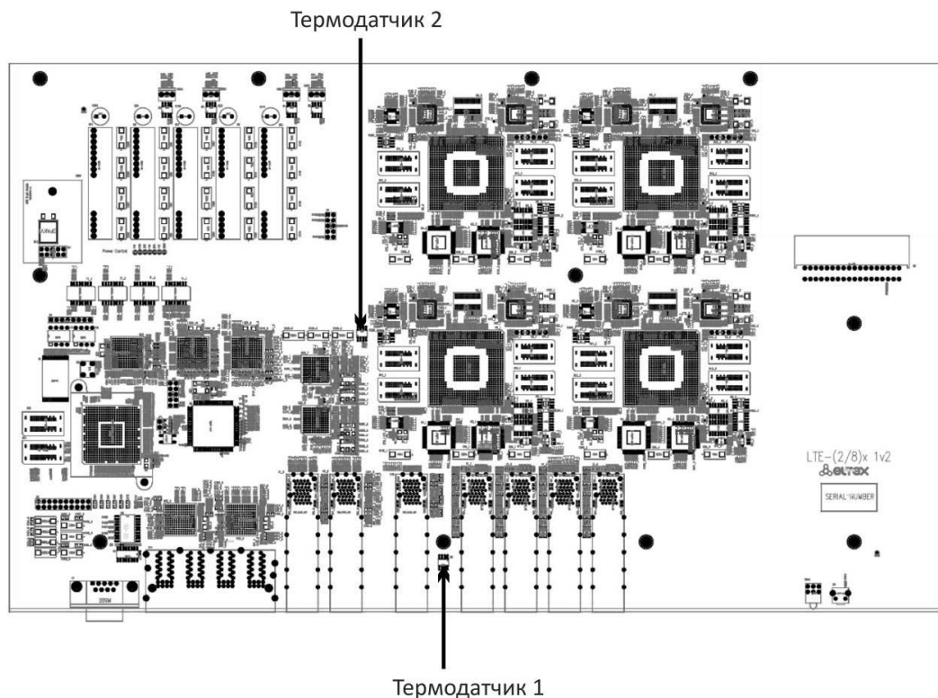
Рисунок 6 – Расположение термодатчиков
