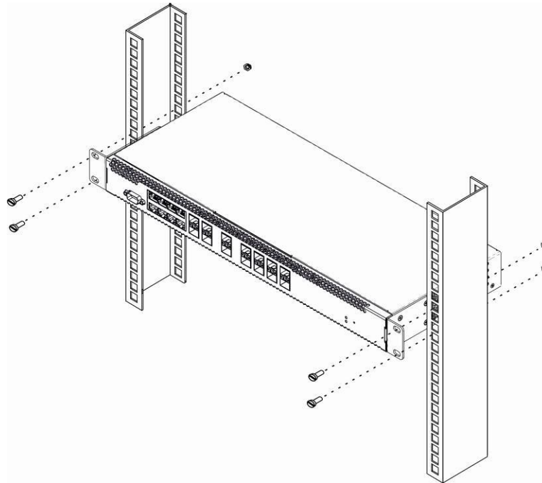
Рисунок 8 – Установка устройства в стойку
