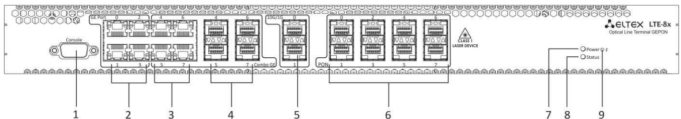
Рисунок 2 – Передняя панель станционного терминала LTE-8X
