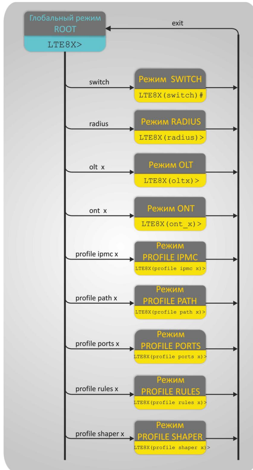
Рисунок 19 – Верхний уровень иерархии режимов команд
