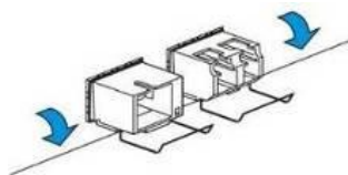
Рисунок 12 – Открытие защелки SFP-трансиверов
