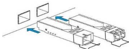
Рисунок 10 – Установка SFP-трансиверов
