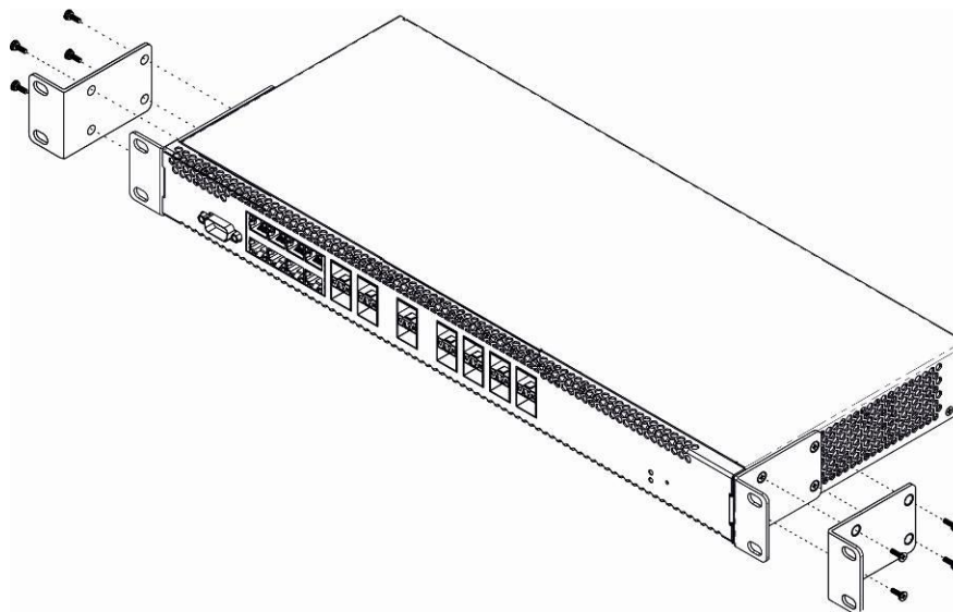
Рисунок 7 – Крепление кронштейнов
