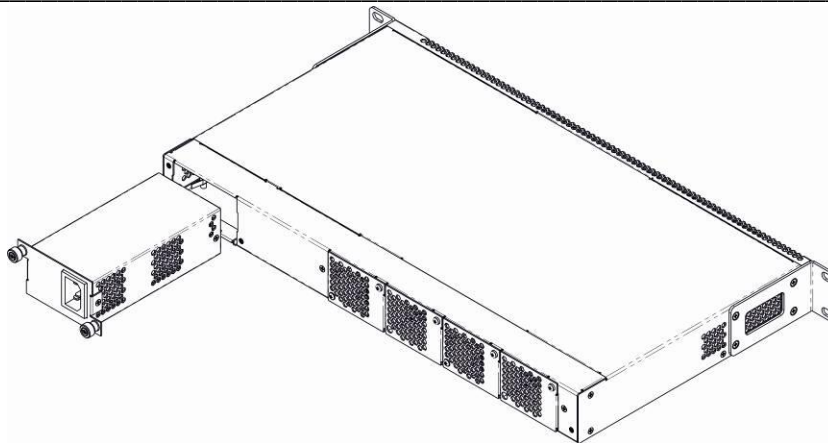
Рисунок 9 – Установка модуля питания.
