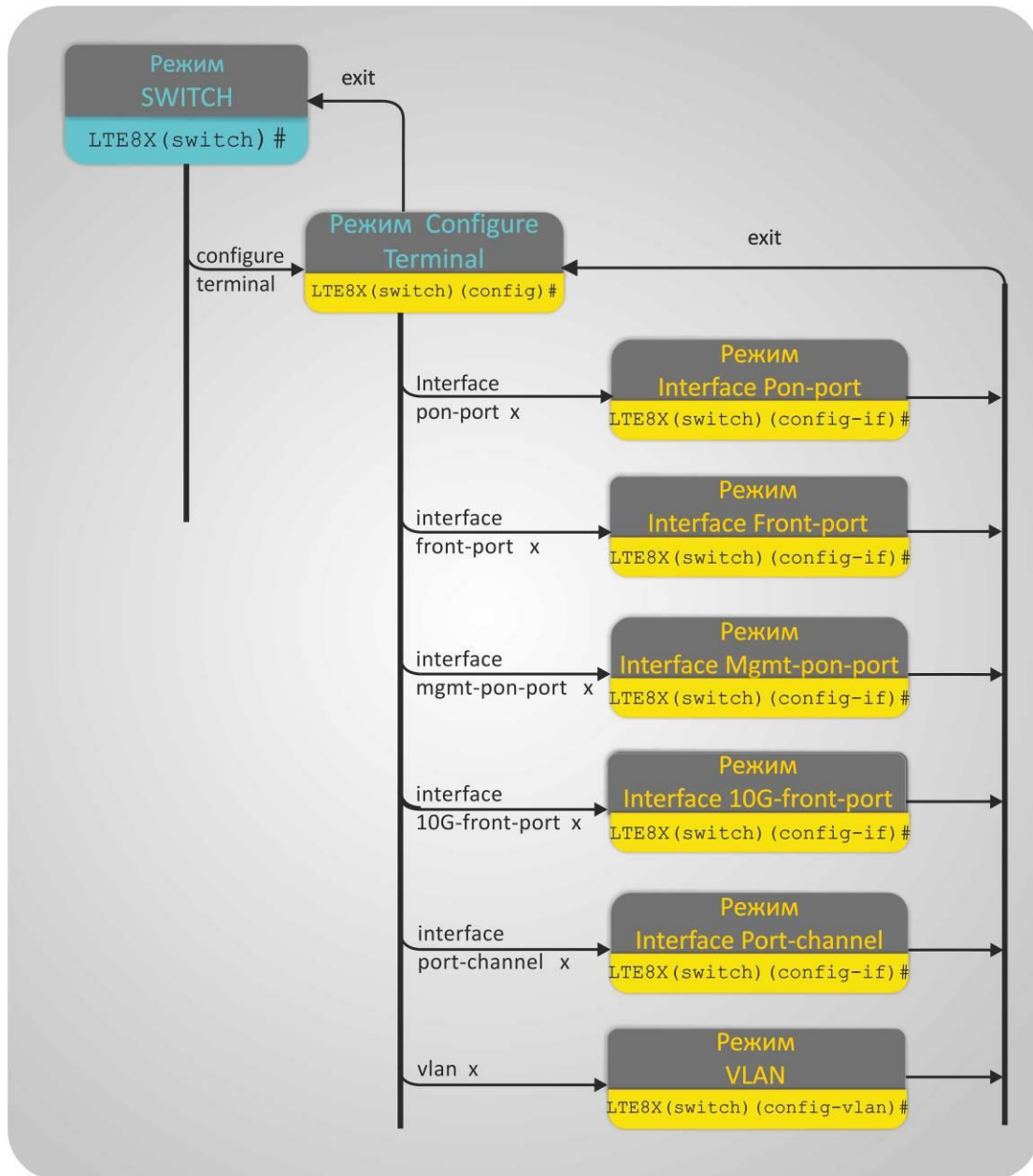
Рисунок 22 – Иерархия командных режимов раздела SWITCH
