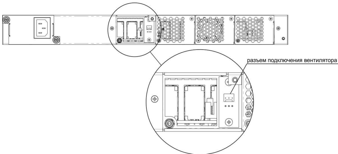
Рисунок 15 – Разъем для подключения вентилятора
