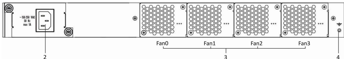
Рисунок 5 – Задняя панель станционного терминала LTE-8X, LTE-2X (AC)
