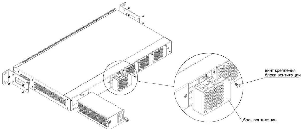
Рисунок 14 – Блок вентиляции. Крепление в корпус
