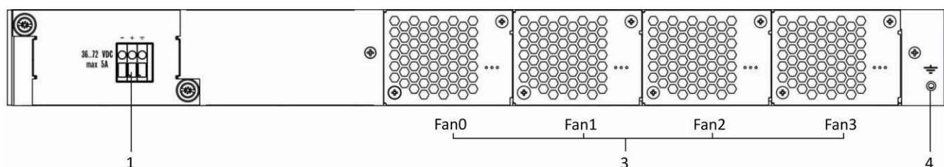
Рисунок 4 – Задняя панель станционного терминала LTE -8X, LTE-2X (DC)
